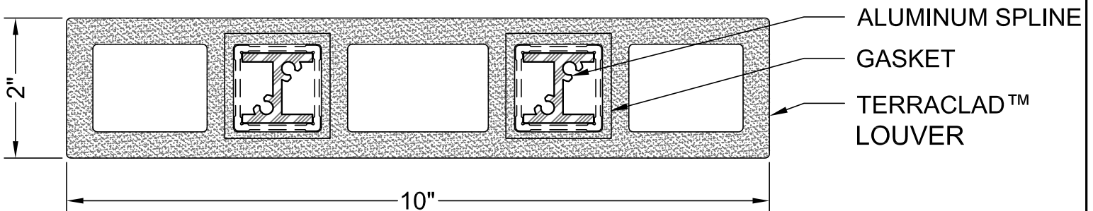
1 2" x 10" LOUVER Scale: 6" = 1'-0"
