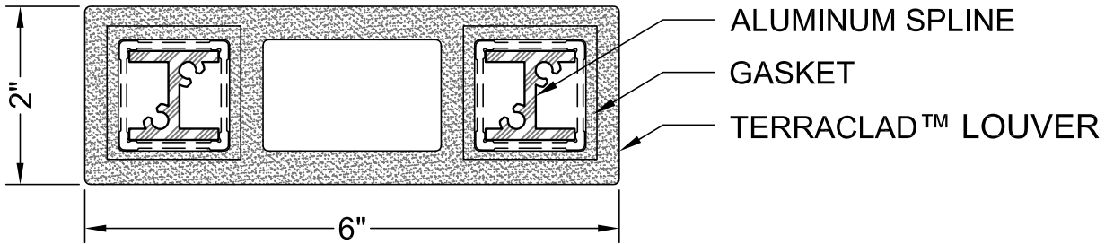
3 2" x 6" LOUVER Scale: 6" = 1'-0"
