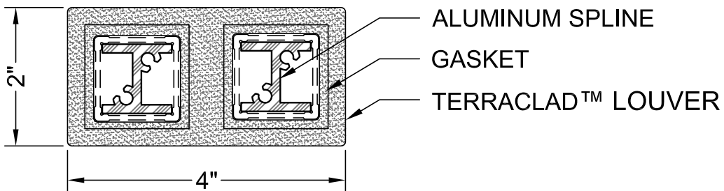
2 2" x 4" LOUVER Scale: 6" = 1'-0"
