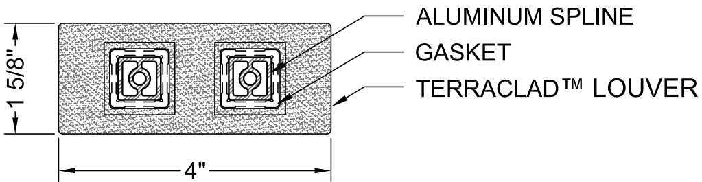
3 1 5/8" x 4" LOUVER Scale: 6" = 1'-0"
