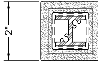
2 2" BAGUETTE Scale: 6" = 1'-0"
